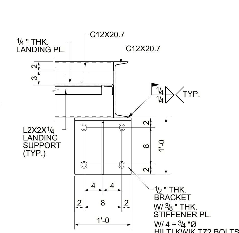
SECTION E1 - E1
