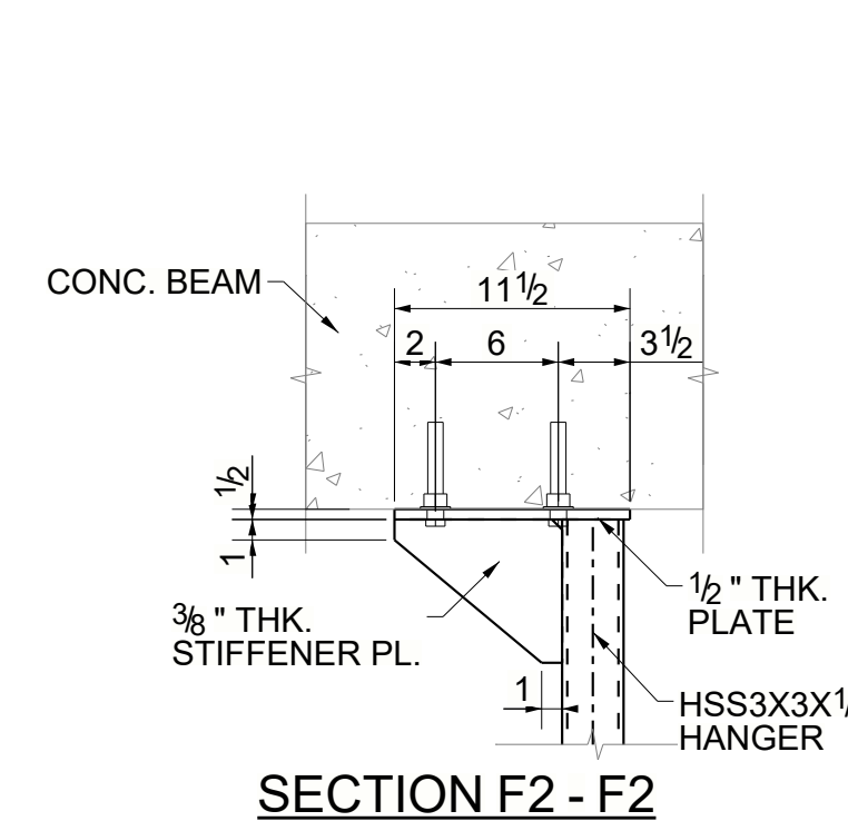
SECTION F2 - F2
