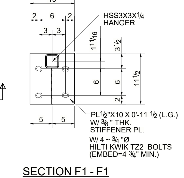
SECTION F1 - F1
